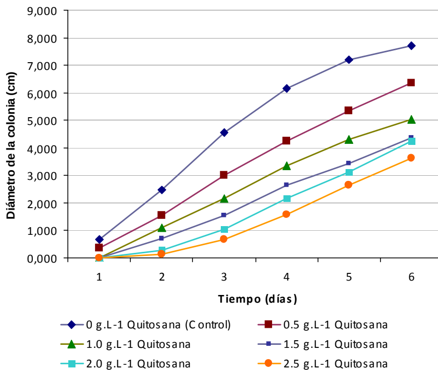
FIGURA 1. Diámetro de las colonias del aislado Pp12 en medio de cultivo V8 con diferentes concentraciones de quitosana. Las barras en cada punto representan los intervalos de confianza para \alpha = 0,05 ./ Colony diameter of Pp12 isolate growing on V8 culture media with different chitosan concentrations. The bars in each point represents the confidence level for \alpha = 0.05 .
