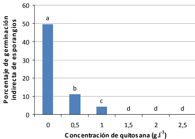
FIGURA 3. Porcentaje de germinación indirecta de esporangios de P. palmivora en diferentes soluciones de quitosana./ Percentage of P. palmivora indirect sporangium germination in different chitosan solutions. ESx= 0.0468.
