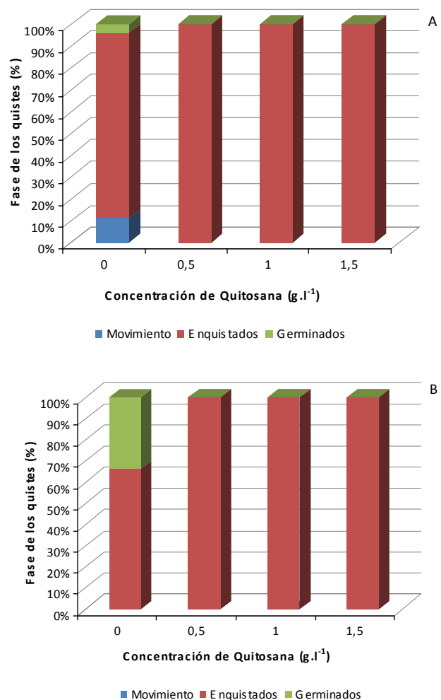
FIGURA 4. Porcentaje de zoosporas de P. nicotianae en diferentes fases (germinación, enquistamiento o movimiento) después de incubarlos durante 60 (A) y 180 (B) minutos con diferentes concentraciones de quitosana./ Percentage of P. nicotianae zoospores at different phases (germination, cyst or movement) after 60 (A) and 180 (B) minutes of incubation with different chitosan concentrations.
