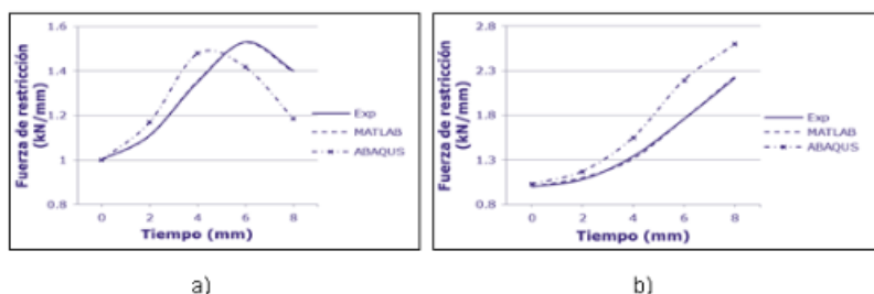
Figura 11. Comparación entre las predicciones con la red neuronal 30-10-1, resultados experimentales y de modelación numérica (ABAQUS). Respuesta: fuerzas de restricción. a) Espécimen experimental HEA160- K128- L70. b) Espécimen experimental HEA160- K45- L30. Fuente: Elaboración propia
