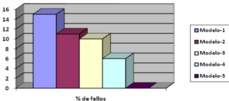
Figura 7. Resultados del entrenamiento por el porcentaje de clasificaciones incorrectas del conjunto de pruebas
