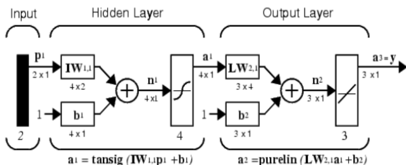
Figura 3. Ejemplo de topología de red Feedforward
