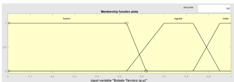
Figura 8. Representación gráfica de la fuzzificación de la variable Estado Técnico, funciones de pertenencia de la variable Estado Técnico, con \gamma_{be} = \alpha_{re} = 0.532 , \delta_{re} = 0.7 , \gamma_{re} = 0.83 , \chi_{re} = 0.95 , \alpha_{me} = 0.84 y \delta_{me} = 0.93 (Estos valores se obtienen como resultado del proceso de agrupación difusa (Fuzzy Clustering) de la información estadística)
