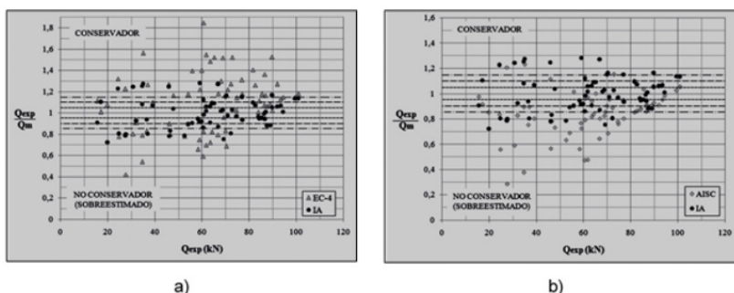
Figura 4. Comparación entre las predicciones con inteligencia artificial y normas internacionales. a) EC-4. b) AISC
