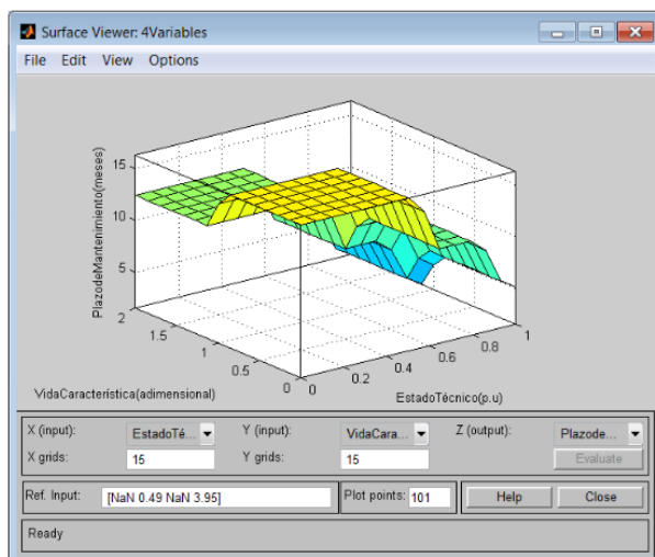
Figura 14. Superficie de comportamiento de la variable del consecuente, en función de la variación de las variables del antecedente estado técnico y vida característica, en el sistema de inferencia de Sugeno para el circuito Las 500
