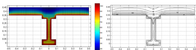
Figura 13. Campo de temperaturas e isoterma de la sección transversal de la viga compuesta para 120 minutos de exposición al fuego. Fuente: Elaboración propia (con imágenes de SuperTempcalc )
