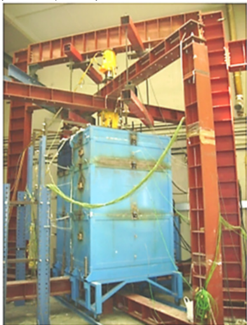
Figura 8. Dispositivo del ensayo de columna restringida en incendio. Fuente: Correia (2011)
