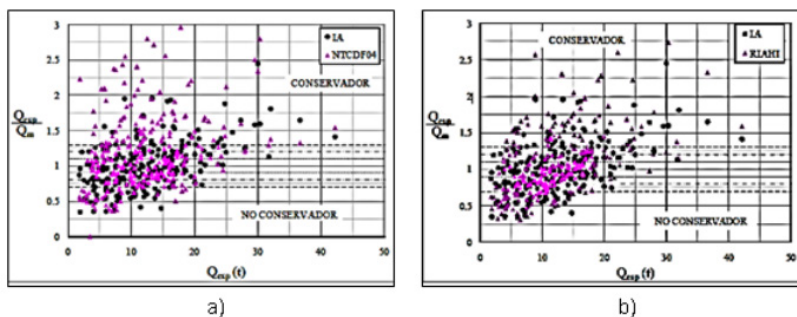
Figura 6. Relaciones Q_{exp}/Q_m para las instancias de la base de datos I en la predicción del cortante de agrietamiento ( V_{agr} ). a) Según IA y GDF (2004). b) Según IA y Riahi et al. (2008). Fuente: Elaboración propia
