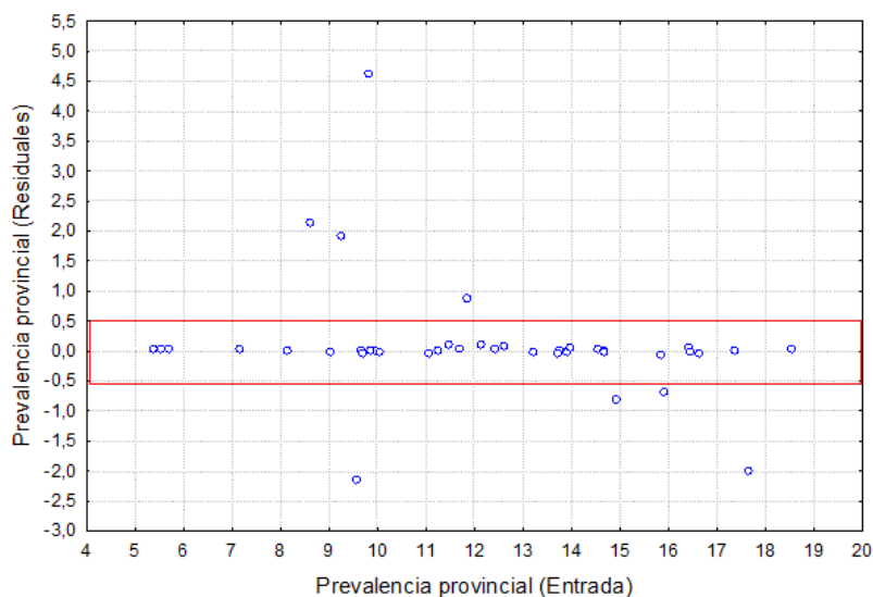
Figura 9. Valor residual de cada prevalencia predecida por el modelo de red neuronal artificial
