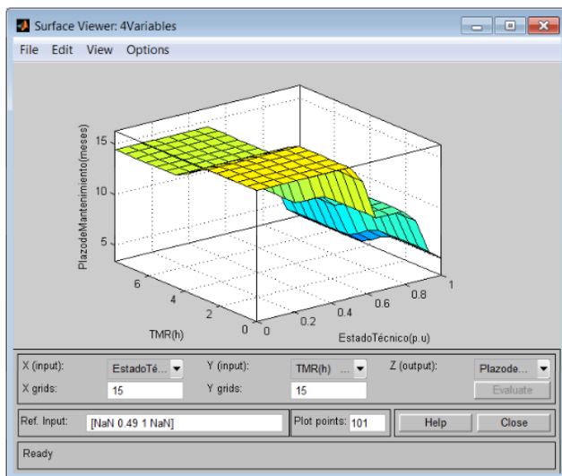
Figura 15. Superficie de comportamiento de la variable del consecuente, en función de la variación de las variables del antecedente estado técnico y TMR, en el sistema de inferencia de Sugeno para el circuito Las 500
