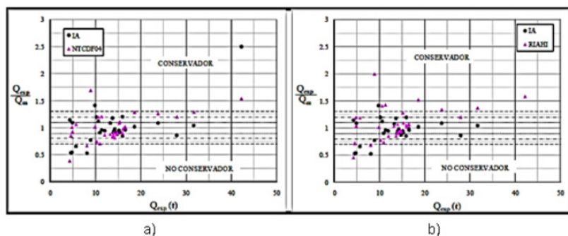
Figura 7. Relaciones Q_{exp}/Q_m para las instancias de la base de datos IV en la predicción del cortante de agrietamiento ( V_{agr} ). a) Según IA y GDF (2004). b) Según IA y Riahi et al. (2008). Fuente: Elaboración propia
