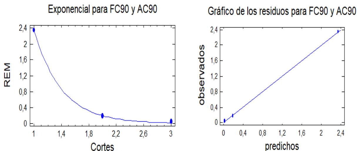
Figura 10. Modelo exponencial ajustado y gráfico de los residuos para el RMS FC90 y AC90 para el período poco lluvioso
