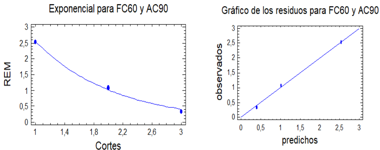
Figura 7. Modelo exponencial ajustado y gráfico de los residuos para el RMS FC60 y AC90 para el período poco lluvioso
