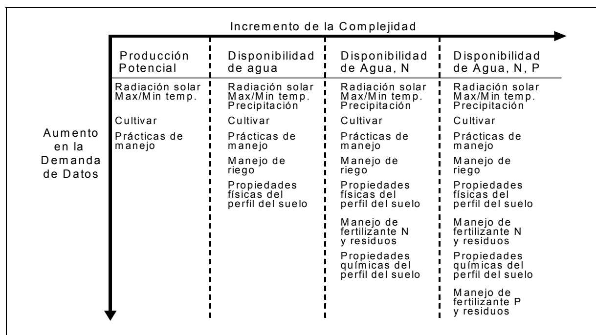
Figura 2. El incremento de los datos necesarios para correr los modelos de simulación de cultivos de DSSAT cuando se incrementa la complejidad de las simulaciones.
